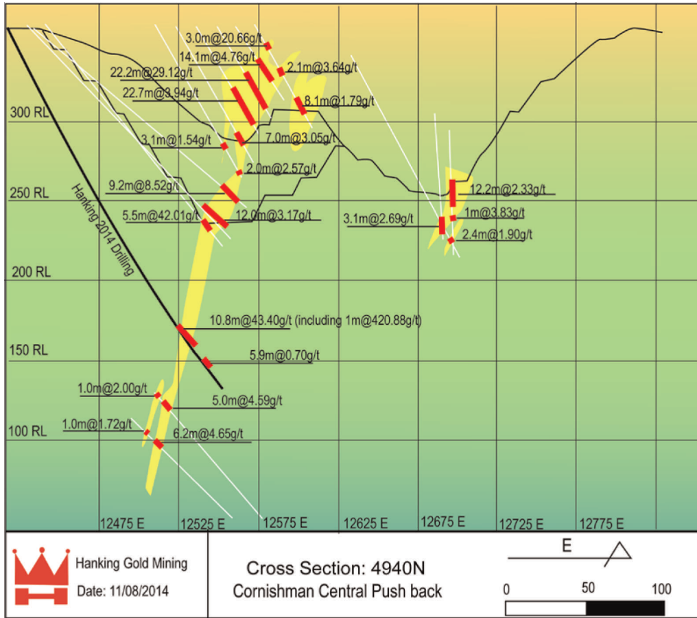
圖1 – Cornishman金礦4940N勘探線剖面圖
